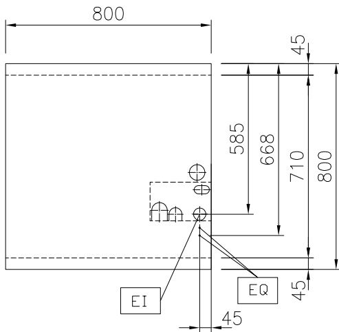
Boven aanzicht
